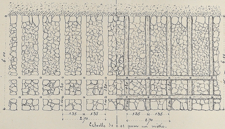
Coupe en travers de la Muraille.
