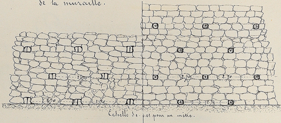
Plan de l'état actuel de la muraille.
