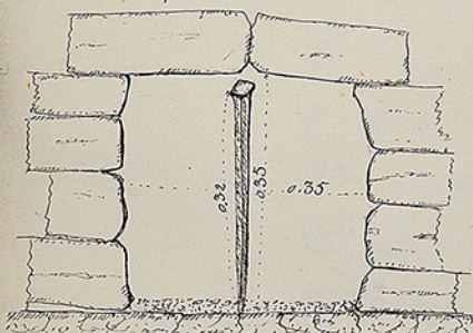
Forme du vide laissé par les poutres et position des clous dans les vides.
