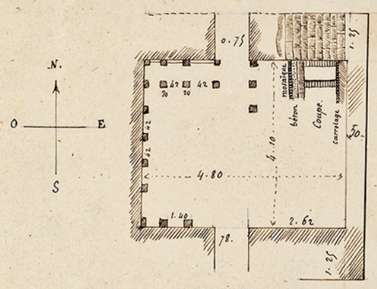
MAISON ROMAINE . Elevation et Plan .
