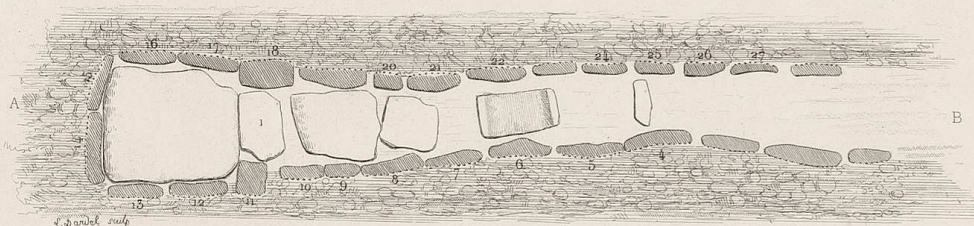
Plan de l'Allée couverte (échelle de 1 centimètre pour 1 mètre)
