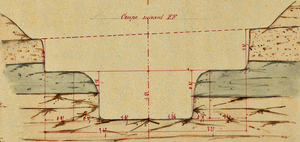
Coupe suivant H.I.
