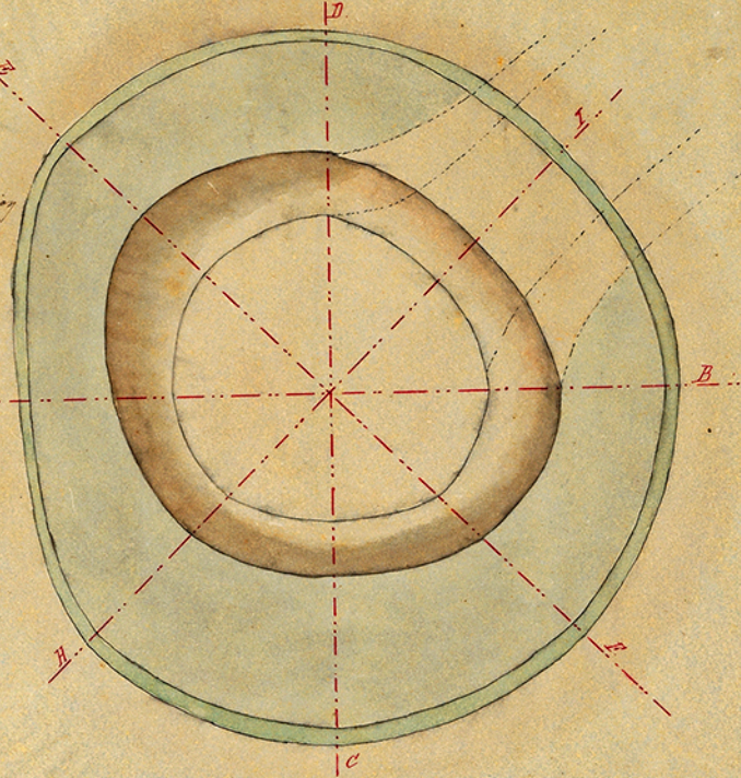
Coupe suivant A.B.
