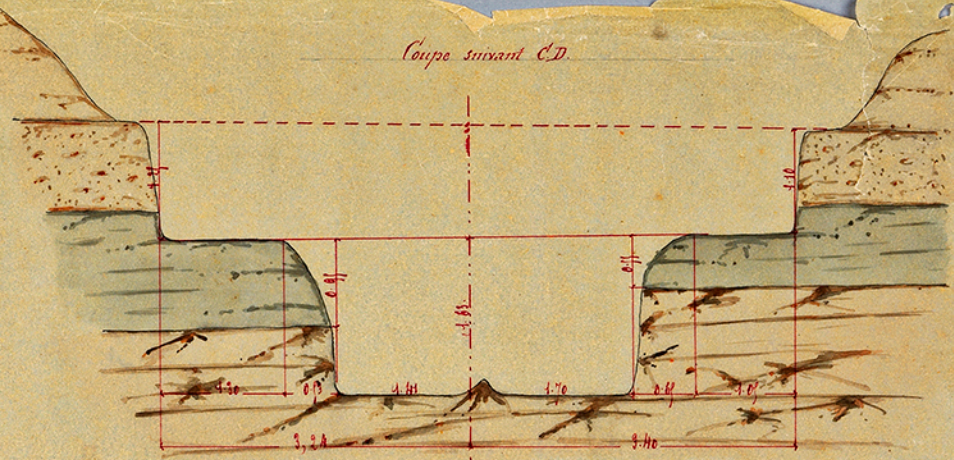
Coupe suivant E.F.
