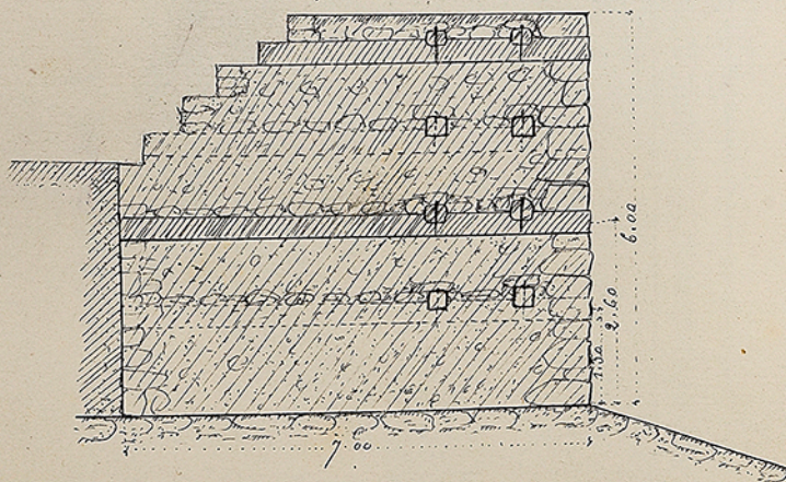
Coupe en travers.
